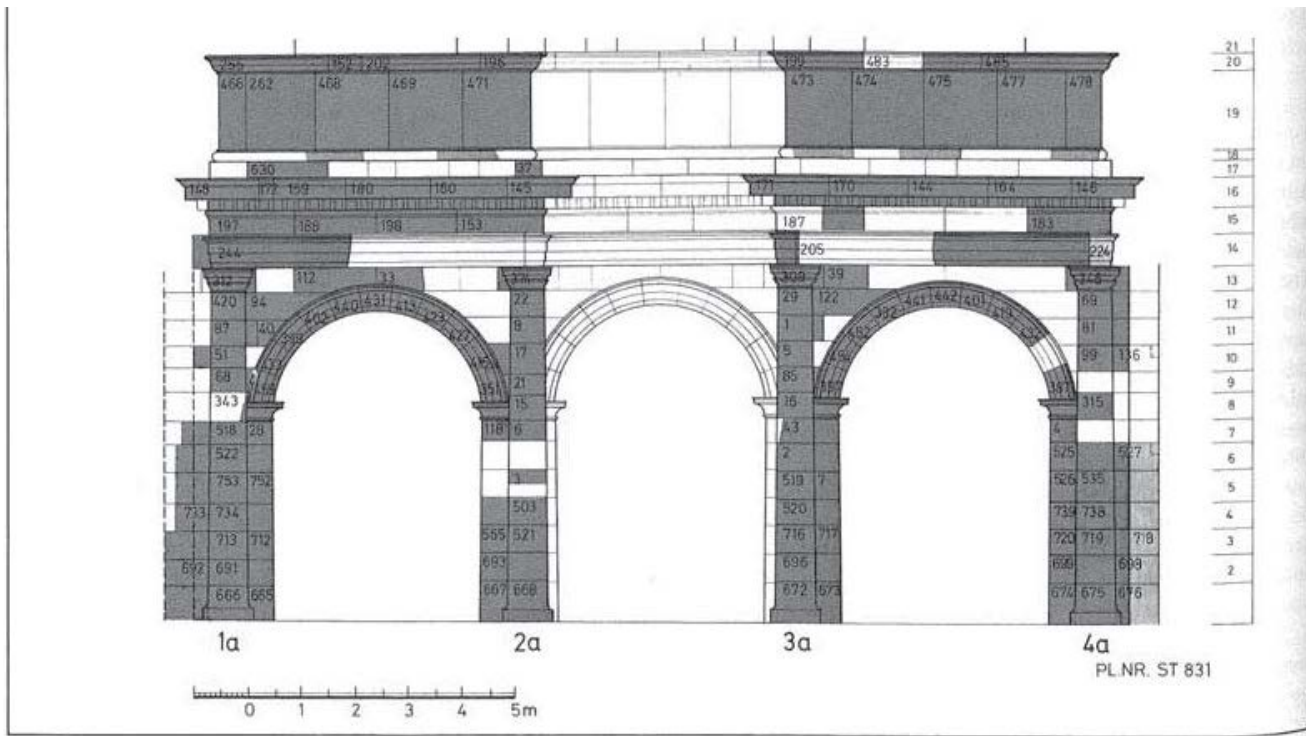
Fig. 3. Porte sud de l'agora, plan de reconstitution de la façade sud montrant les éléments originaux intégrés dans l'élévation. (Fr. Lang, 1984 p. 24 fig. 2).
