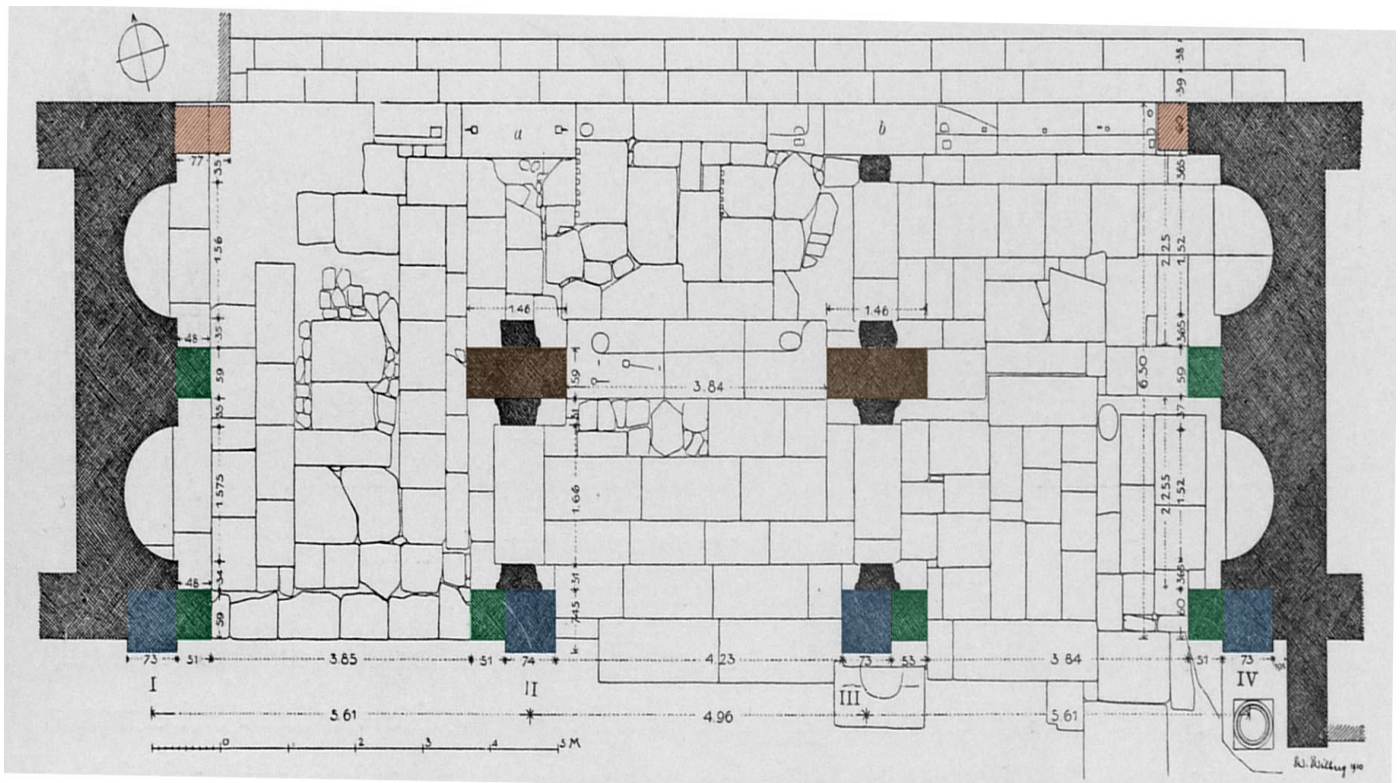
Fig. 7. Porte sud de l'agora, plan des fondations de la porte selon les mesures prises au début du XXe s. Les portions colorées renvoient à des éléments architecturaux de même dimensions : blocs parallélépipédiques centraux (146 x 59 cm, brun); piles de façade soutenant entablement (74x74 cm, bleu; pilastres adossés (48-51 x 59 cm, vert) ; deux fondations parallèles au nord; supposées ? (77 x ca. 60 cm, orange). B. Wilber 1923 FiE 3, p. 41.
