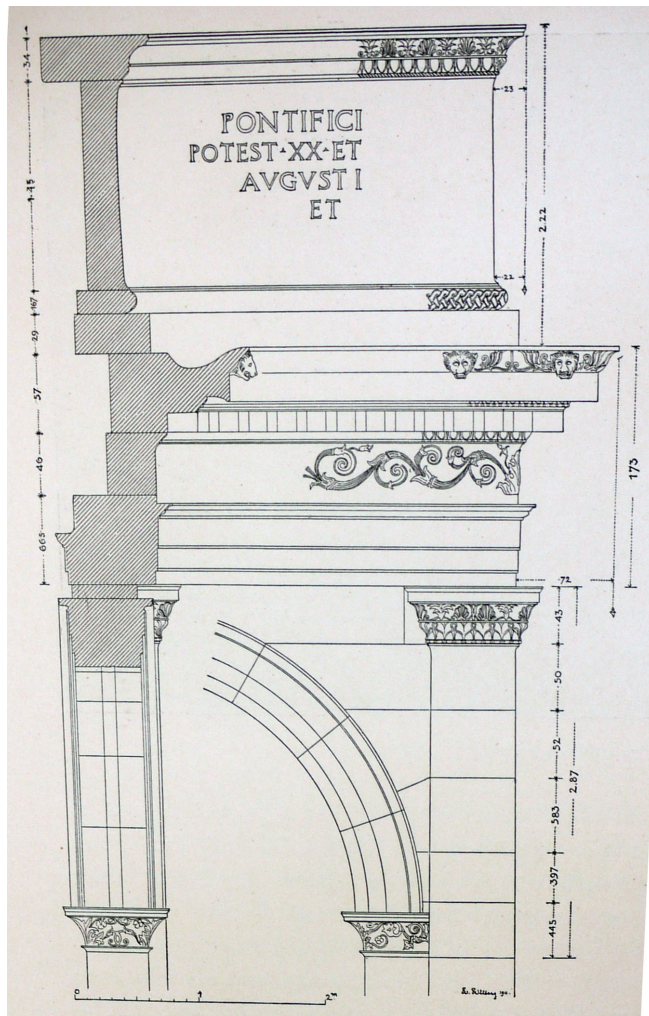
Fig. 13. Porte sud, coupe médiane de l'édifice avec indication de hauteur des éléments d'élévation : piliers de façade sud, pilastres portant les arcs; linteaux de portes longitudinales (B. Wilber 1923 FiE , p. 54, fig. 87).
