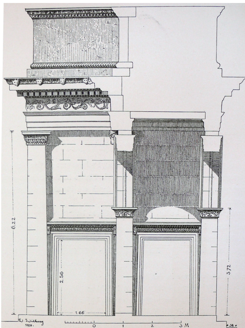
Fig. 8. Porte sud de l'agora, coupe médiane de l'édifice avec indication de hauteur des éléments d'élévation : piliers de façade sud, pilastres portant les arcs; linteaux de portes longitudinales (B. Wilber 1923 FiE p. 54 fig. 87).
