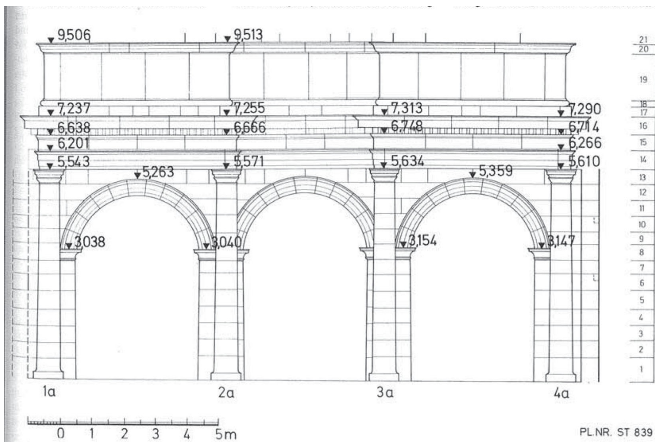
Fig. 4. Porte sud de l'agora, plan intégrant les côtes d'élévation en vue de la reconstruction de l'édifice (Fr. Lang 1984 p. 29).
