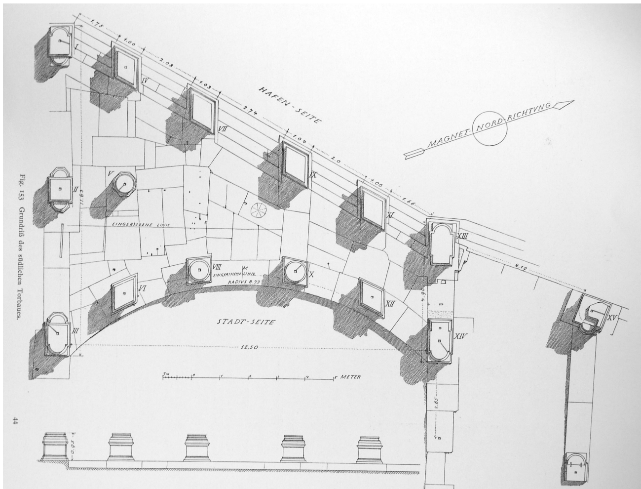
Fig. 38. Planimétrie de la porte sud du port (G. Niemann FiE1923 Torbau am Hafen S , fig. 153)
