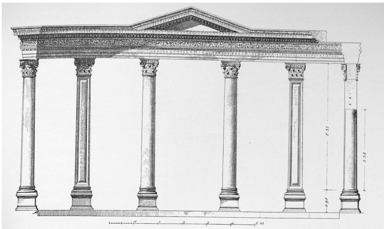
Fig 39. Reconstitution de l'élévation de porte sud du port. Façade orientale tournée vers la ville (G. Niemann FiE1923 ,Torbau Hafen S , fig. 162 p. 177).
