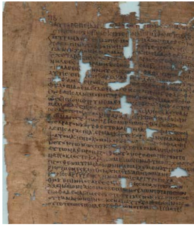
stretchlim
