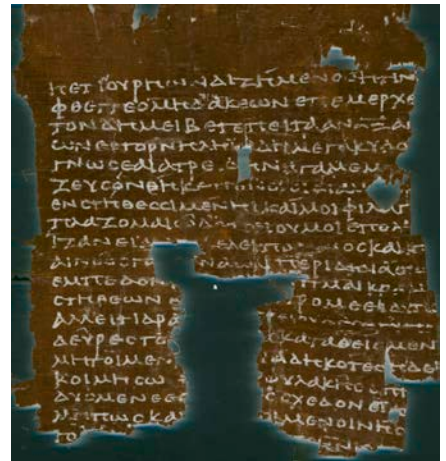
neglsv
