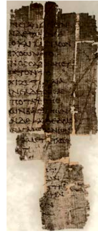
histeq
